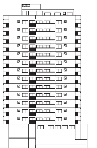
FACHADA TRAVESSA LÓCIA ESC.: 1/200
