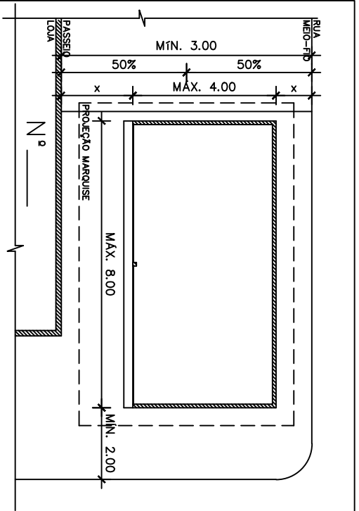
02 PLANTA BAIXA ESCALA 1:75
